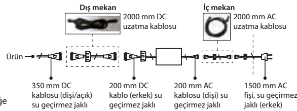
Dış mekana dayanıklı güç kaynağı (IP67)
