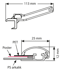
Profil açma aparatı UYUP047000
