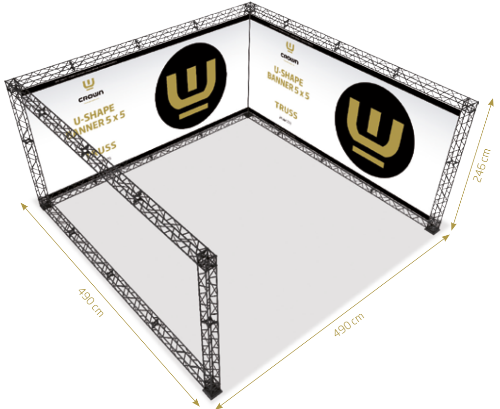
Truss U-Şekil 5 x 5 Stand Sistemi
